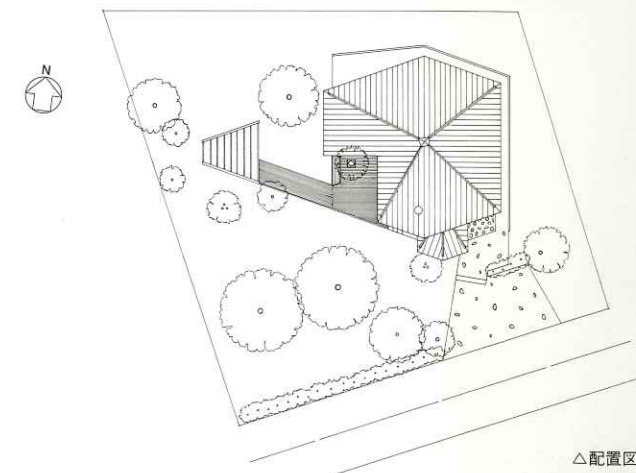
△配置図
